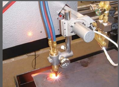
《 하나의 산소 가스토치 》
